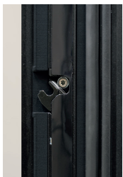
Der Verschluss mit pferdekopfförmiger Verriegelung im Rahmen
